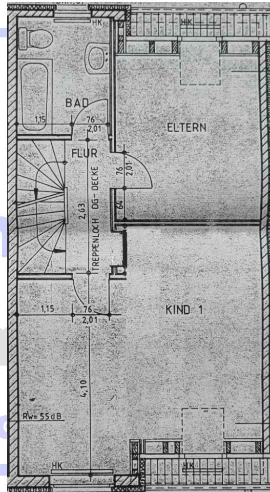
Obergeschoss
