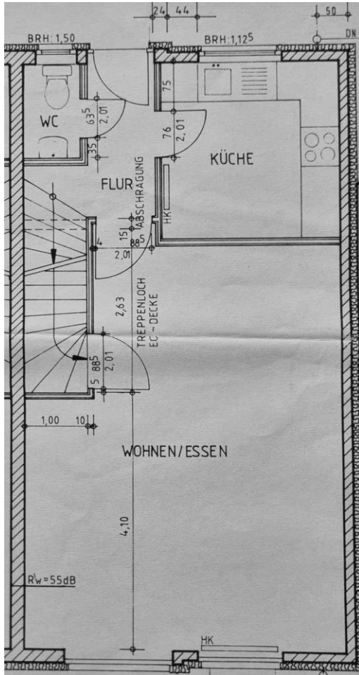
Erdgeschoss
